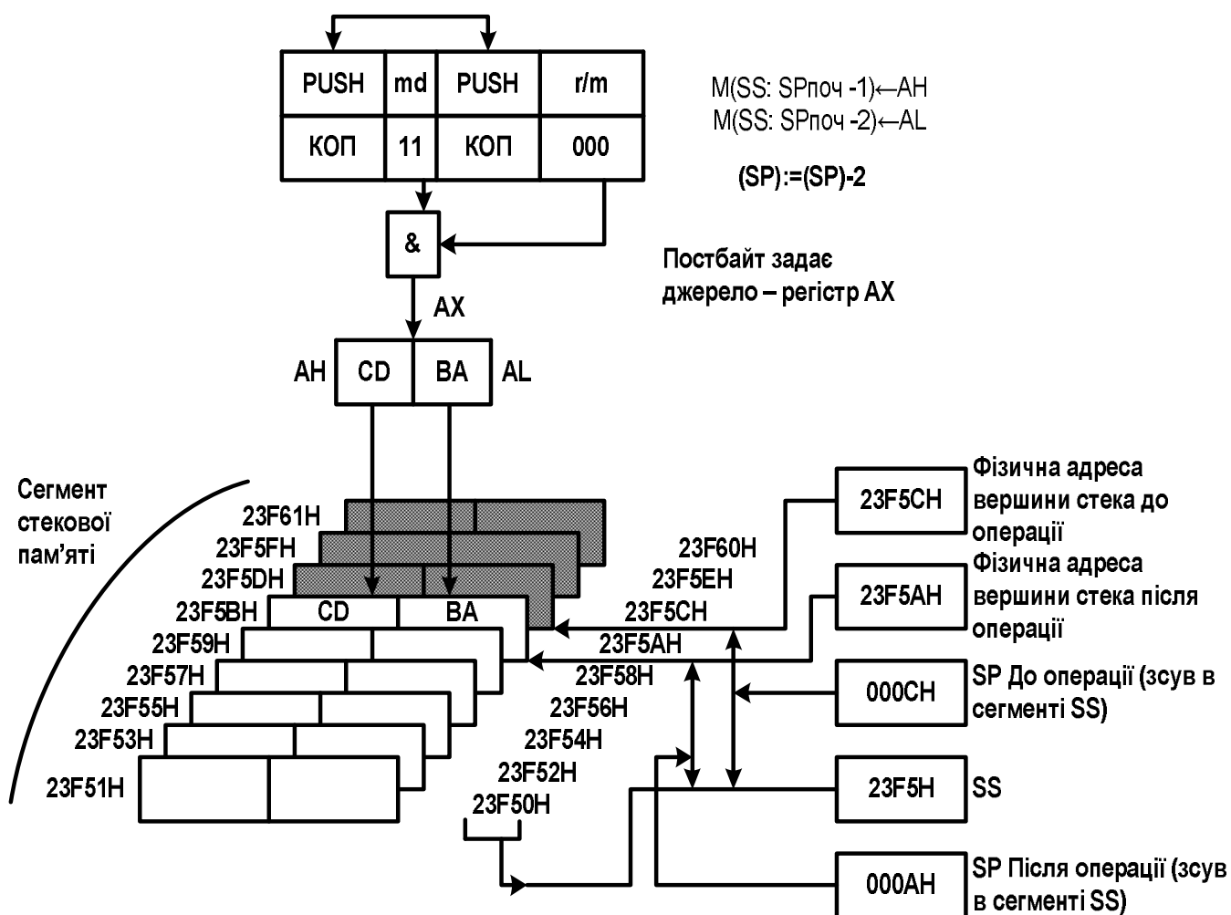
Рисунок 7.11 – Стекова адресація
