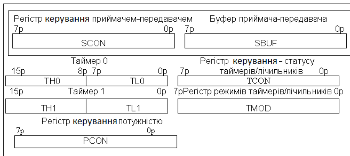
Рисунок 4.5 – Програмна модель МК51
