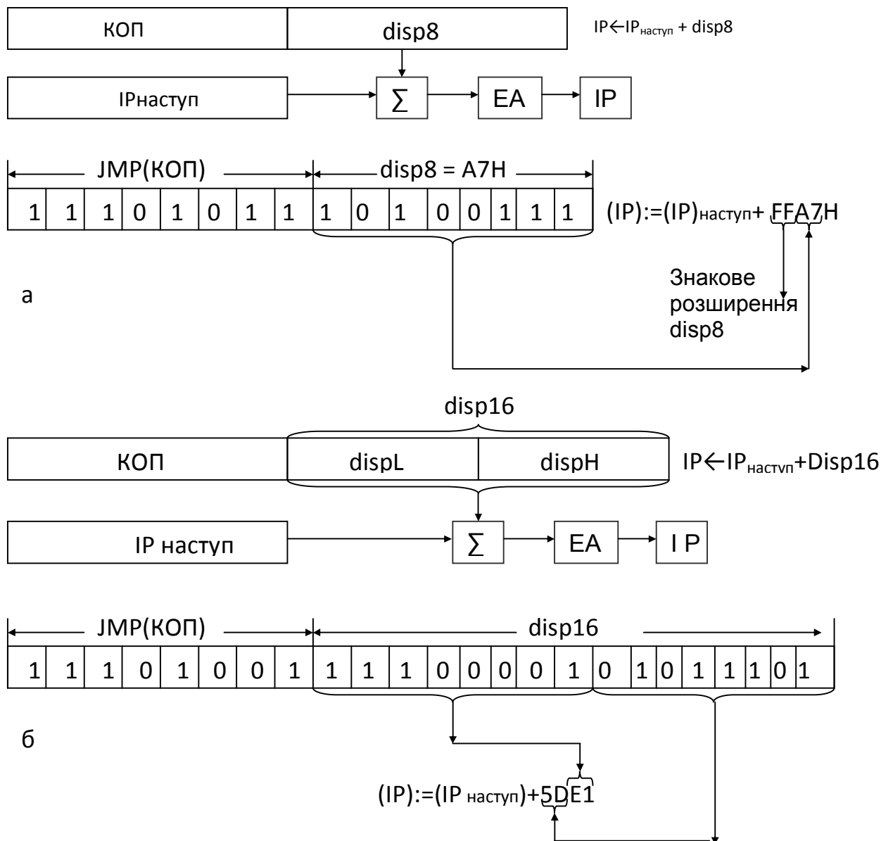
Рисунок 7.12 – Відносна адресація
