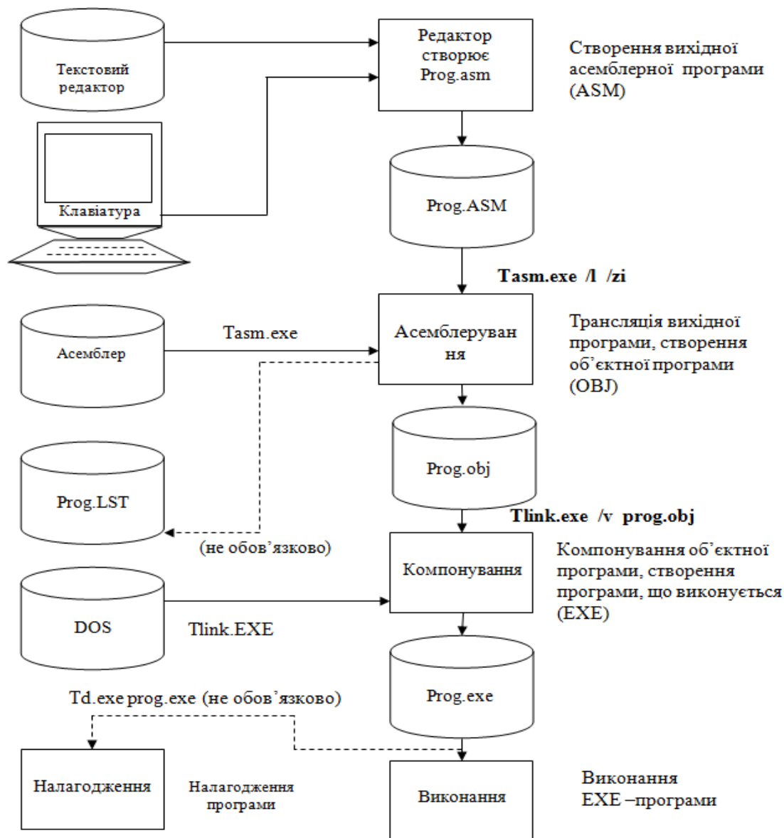
Рисунок 5.1 – Схема асемблювання, компонування, налагодження і виконання програми
