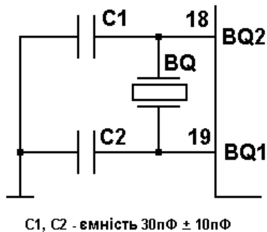
Рисунок 3.6 – Схема підключення кварцового резонатора
