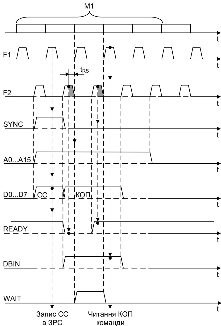
Рисунок 3.13 – Часові діаграми роботи МП-ра i8080 для МЦ «читання коду операції команди»
