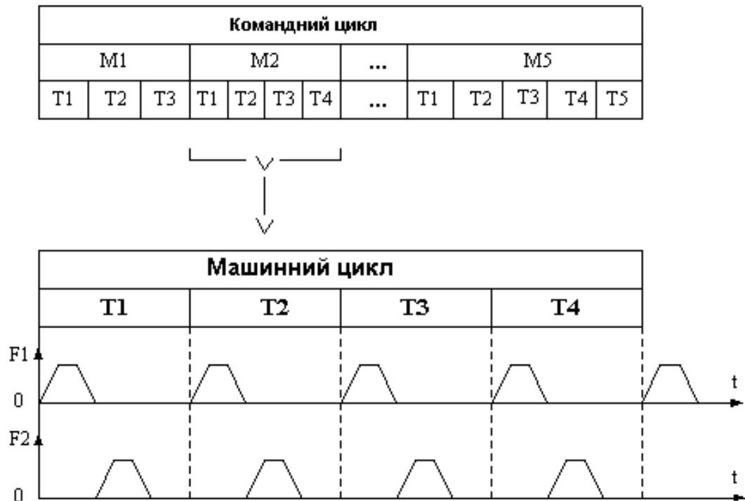
Рисунок 6.8 – Формат командного циклу МП i8080
