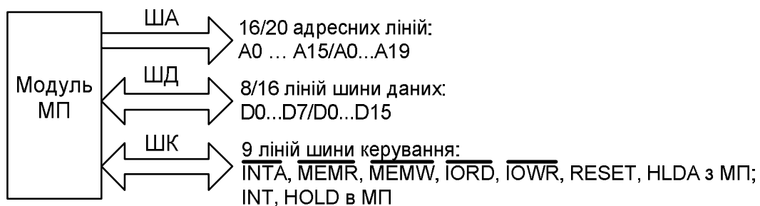
Рисунок 3.11– Структурна схема системи з 3 шинами
