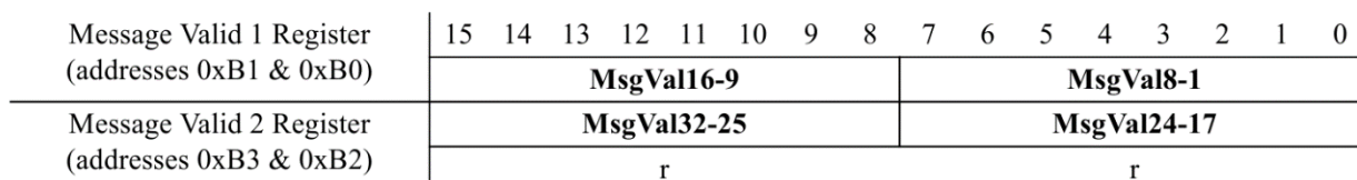
Рисунок 11.36 – Message Valid 1 Register
