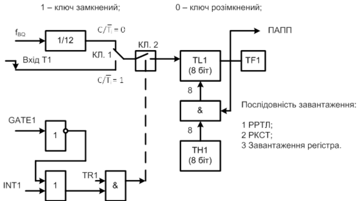
Рисунок 3.2 – Спрощена структурна схема таймера/лічильника 1 в режимі 2
