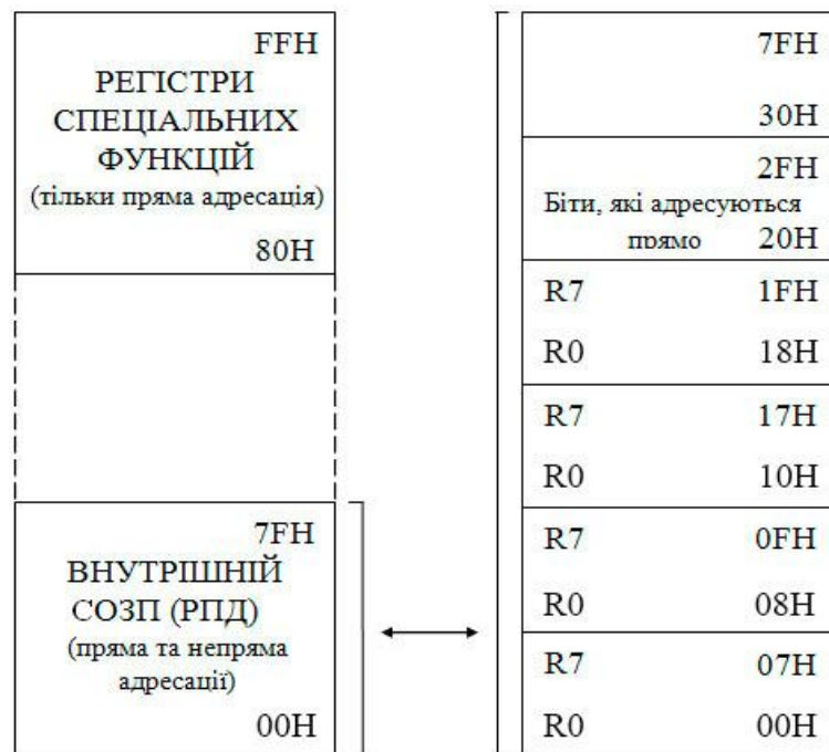
Рисунок 7.6 – Адресний простір внутрішньої статичної пам'яті даних (SRAM) та регістрів спеціальних функцій (PCF)
