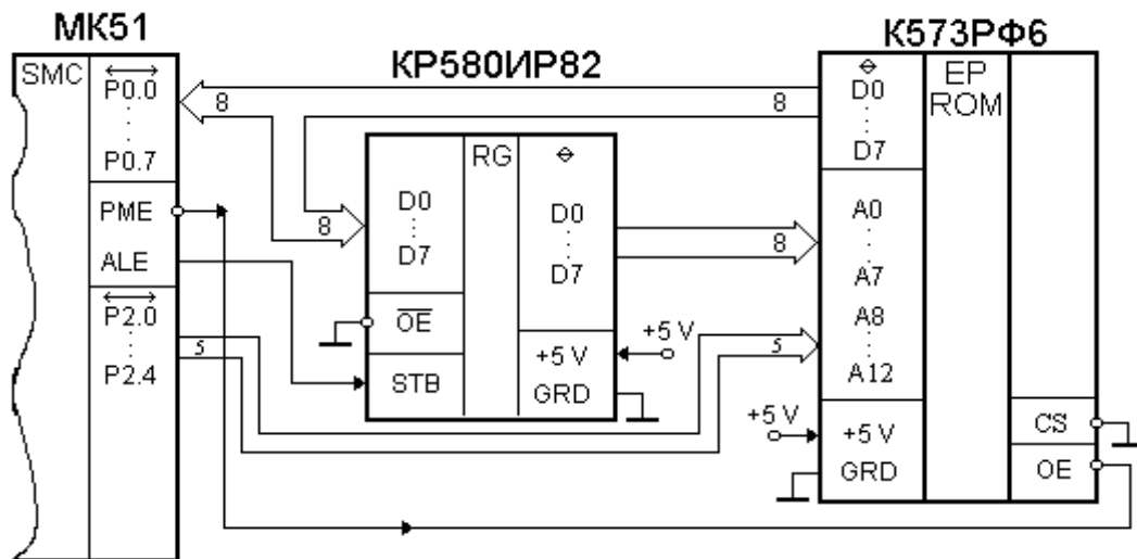
Рисунок 7.10 – Підключення ЗПП (8 Кбайт) до МК–51
