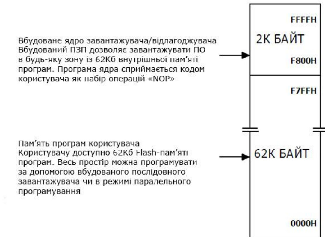
Рисунок 7.13 – Карта розподілу Flash-пам'яті програм в нормальному режимі роботи
