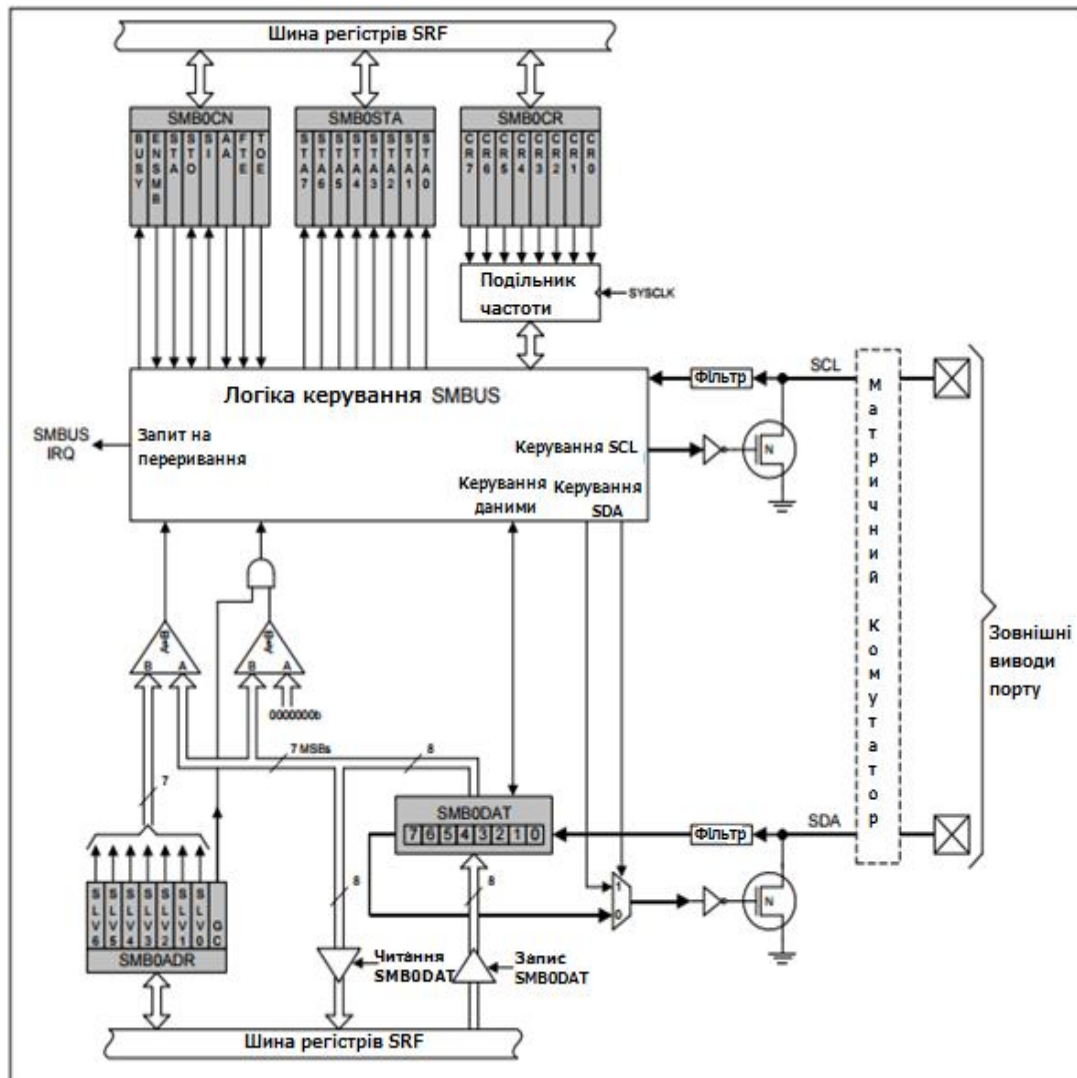
Рисунок 6.17 – Функціональна схема контролера послідовного інтерфейсу SMBus0
