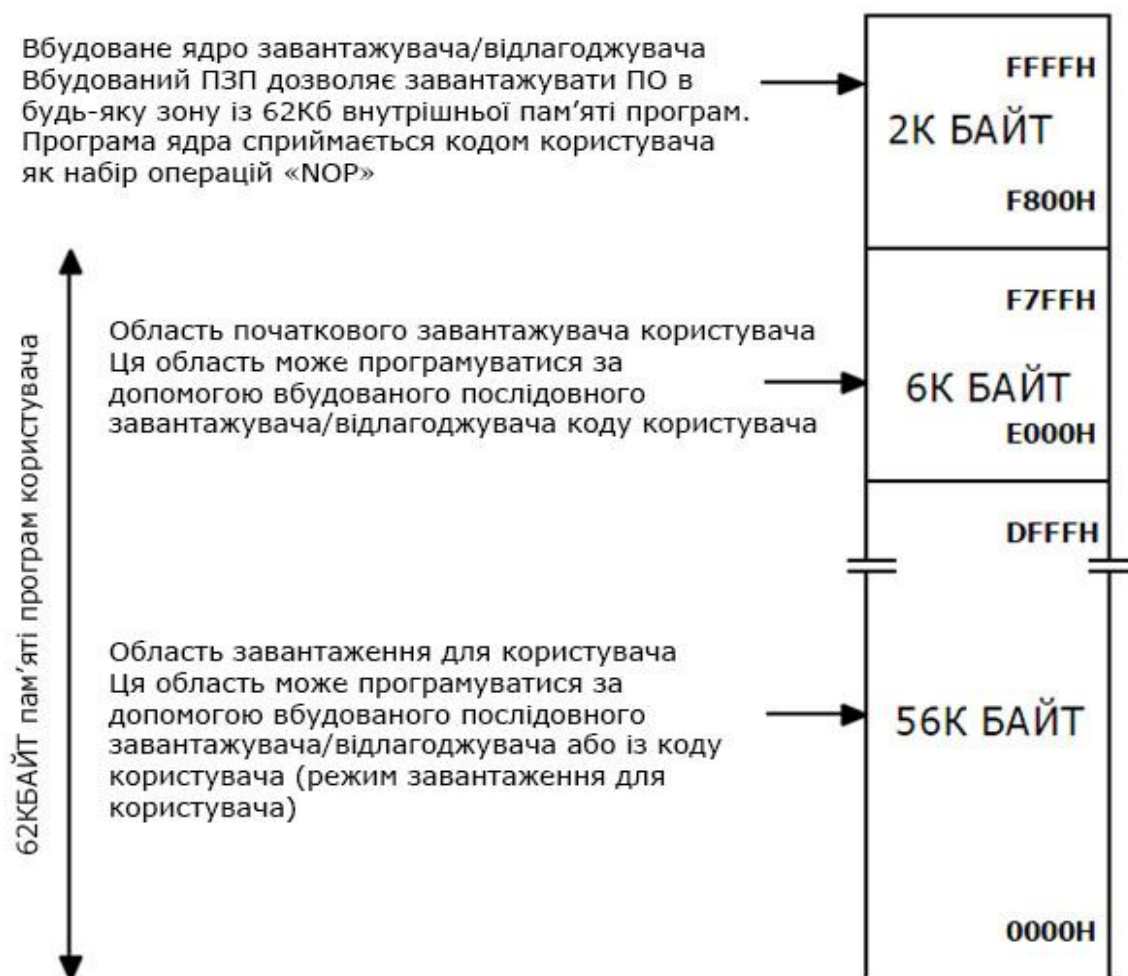
Рисунок 7.14 – Карта Flash-пам'яті в режимі завантаження ПЗ
