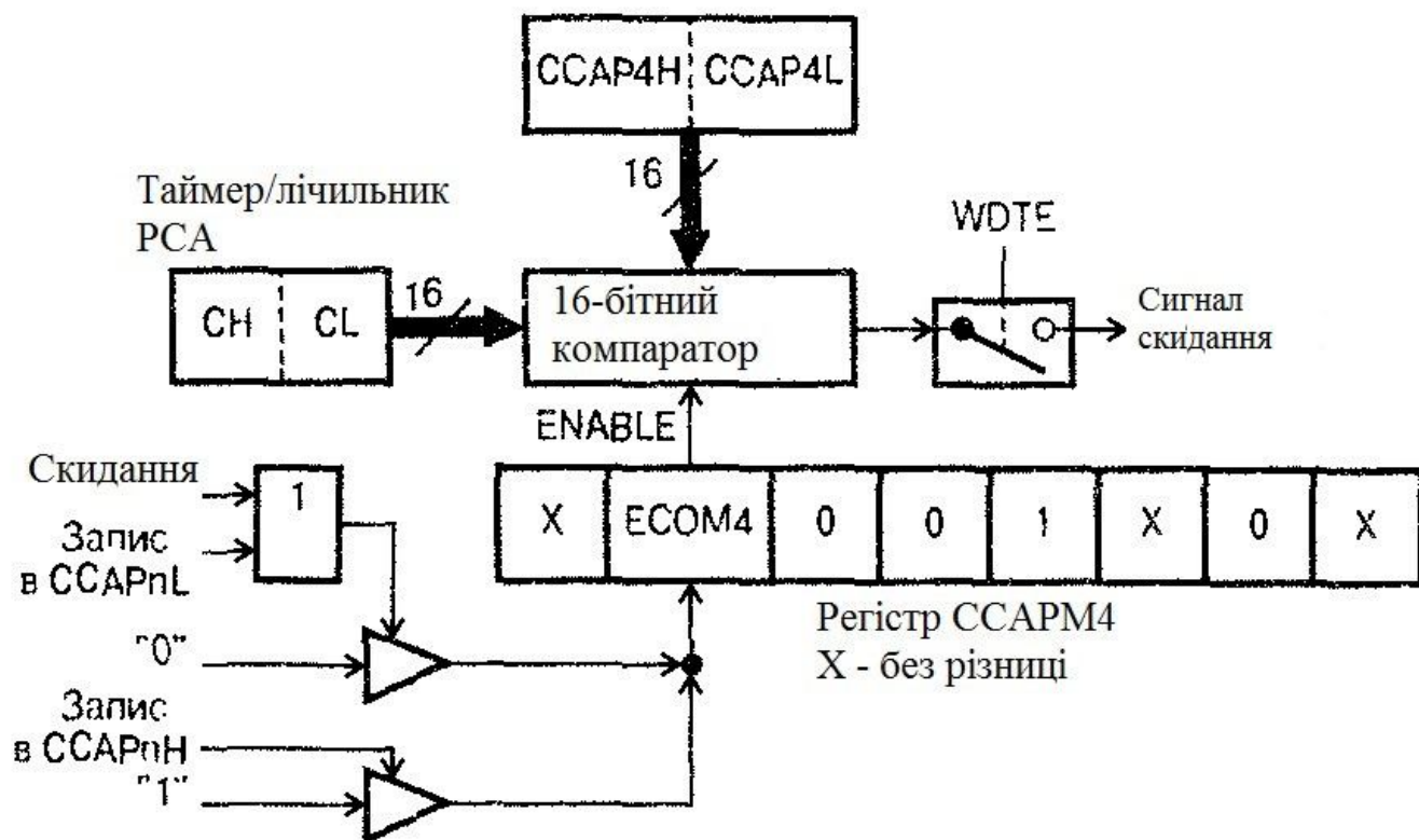
Рисунок 3.9 – Спрощена структура таймера PCA в режимі вартового таймера
