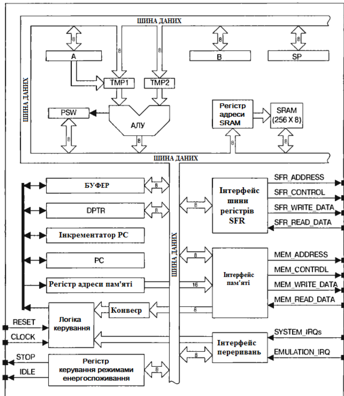
Рисунок 1.1 – Структура ядра CIP-51
