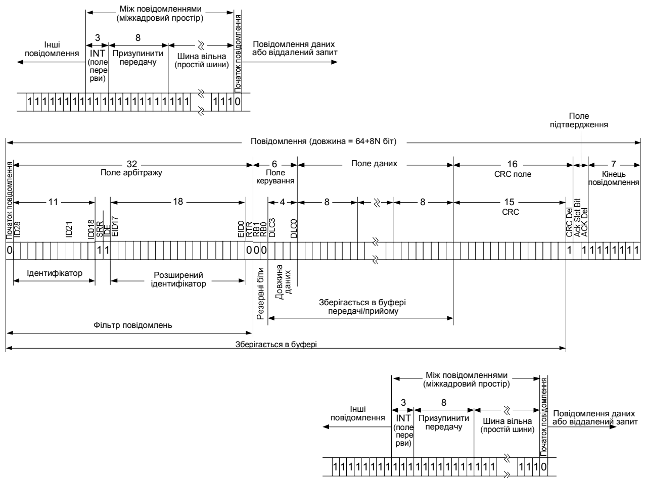
Рисунок 11.2 – Розширене повідомлення
